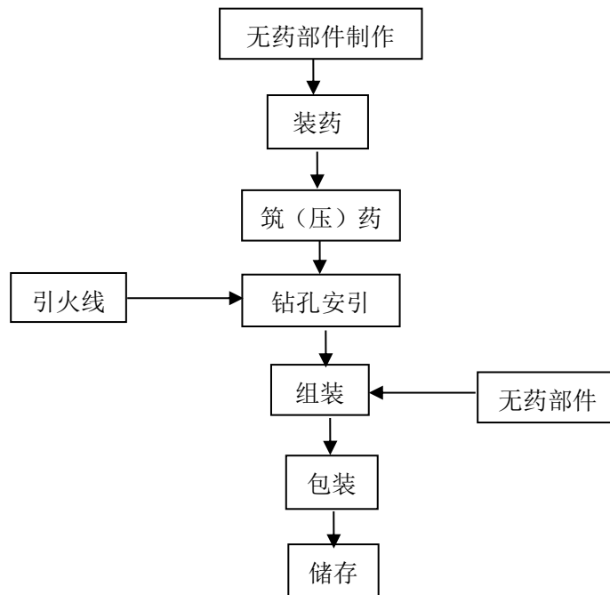
图 2-4-2 旋转类（无固定轴）生产工艺流程图
